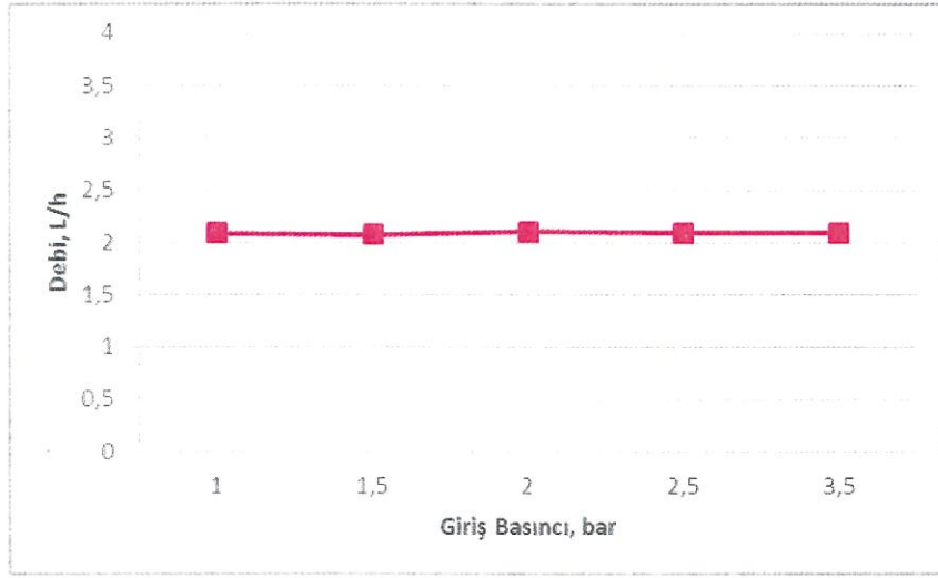
Şekil 3. Dripnet 20010 2.0 l/h, 1mm et kal. 50 cm dam. aralıklı borulara ait basınç debi değişimi
