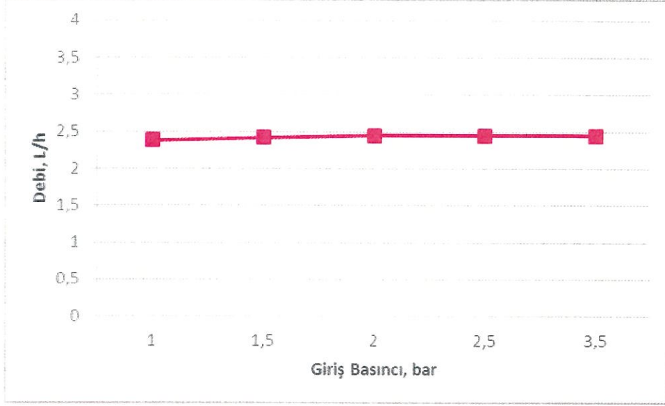
Şekil 3. Uniram 20010 2.3 l/h, 1mm et kal. 60 cm damlatıcı aralıklı borulara ait basınç debi değişimi
